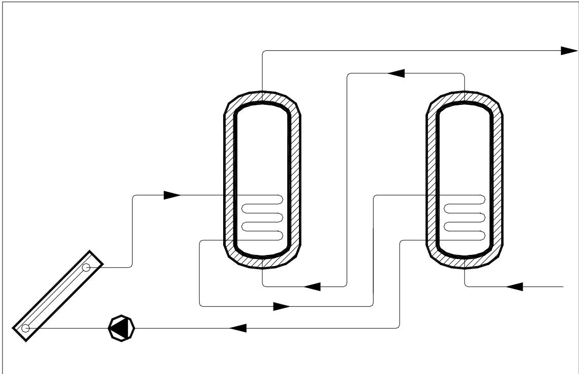
FIG. 20a CONEXION EN SERIE INVERTIDA CON EL CIRCUITO DE CONSUMO
